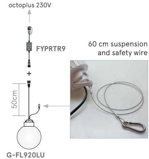
FL920LU G-FL920LU
